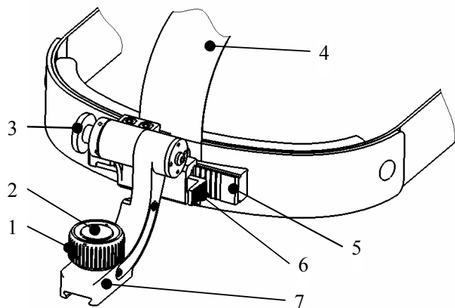
1 — фиксатор; 2 — кнопка; 3 — кнопка; 4 — ремешок; 5 — направляющая; 6 — кнопка; 7 — кронштейн
